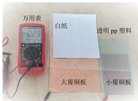
图 2 实验装置图
